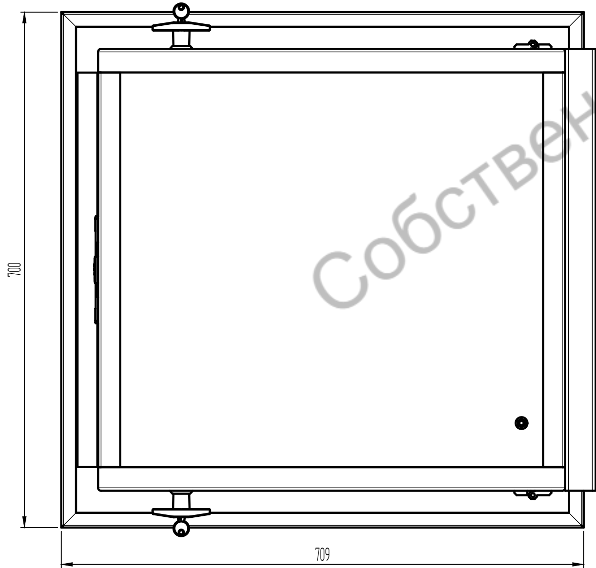
Вид снизу
