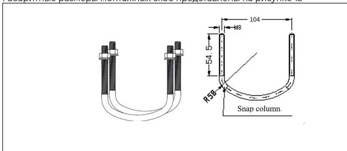
Рисунок 11 – габаритные размеры монтажных скоб
