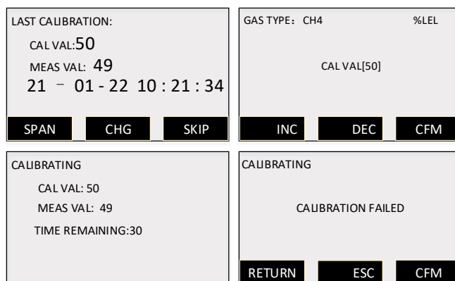
Рисунок 33: калибровка чувствительности
