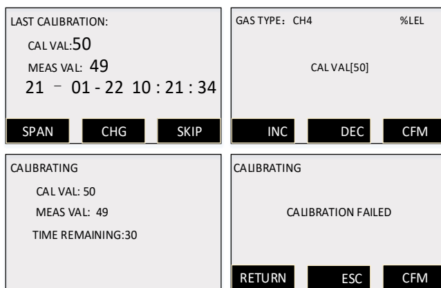
Рисунок 33: калибровка чувствительности
