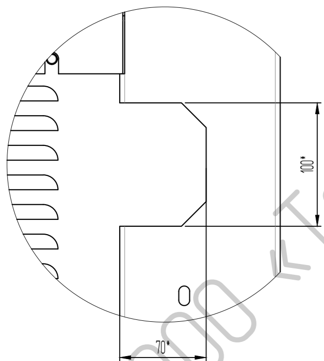
Вид Ж, 2 места (1:3)
