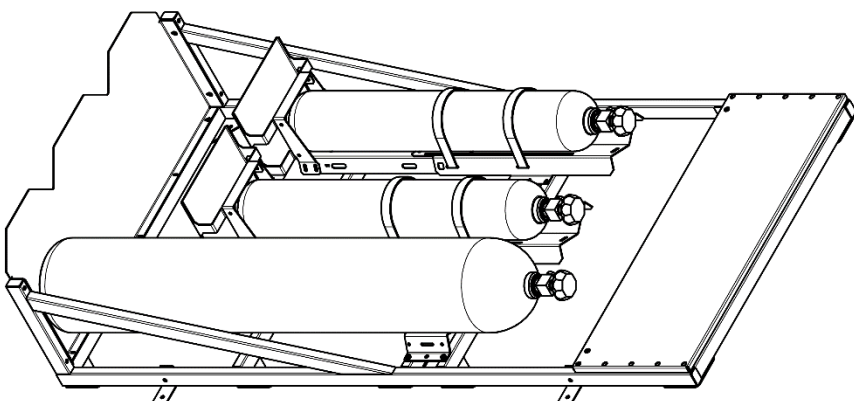
Баллонная стойка, модель ТДМ-СБМ-03 с установленным баллонным адаптером ТДМ-АБУ-5-10
