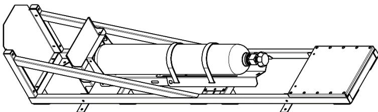
Баллонная стойка, модель ТДМ-СБМ-01 с установленным баллонным адаптером ТДМ-АБУ-5-10
